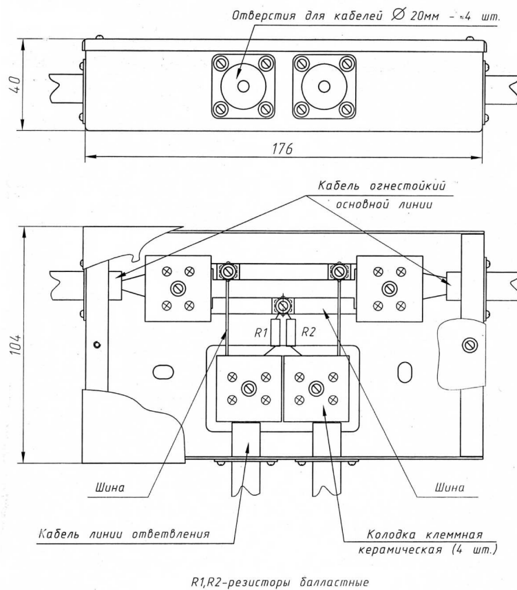
Рис. 1 Схема підімкнення коробки вогнестійкої розподільчої
