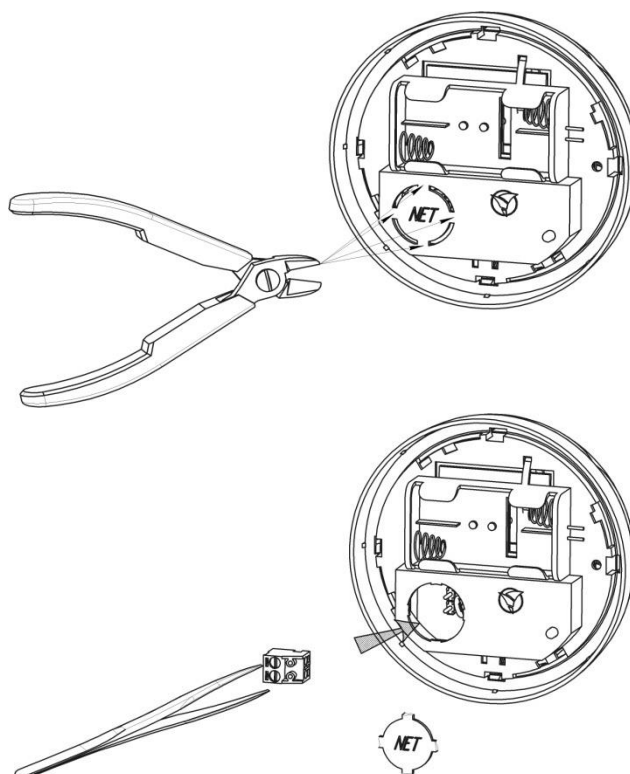
Малюнок 9 - Вилучення заслінки та встановлення клемника (роз'єму) в сигналізатор
