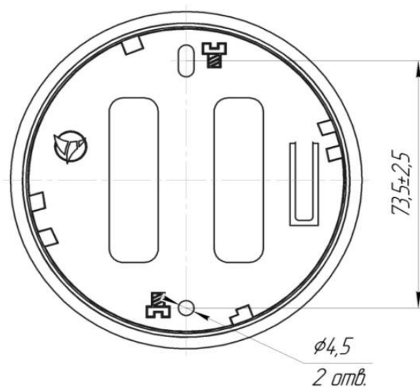
Малюнок 6 - Основа. Зовнішній вигляд
