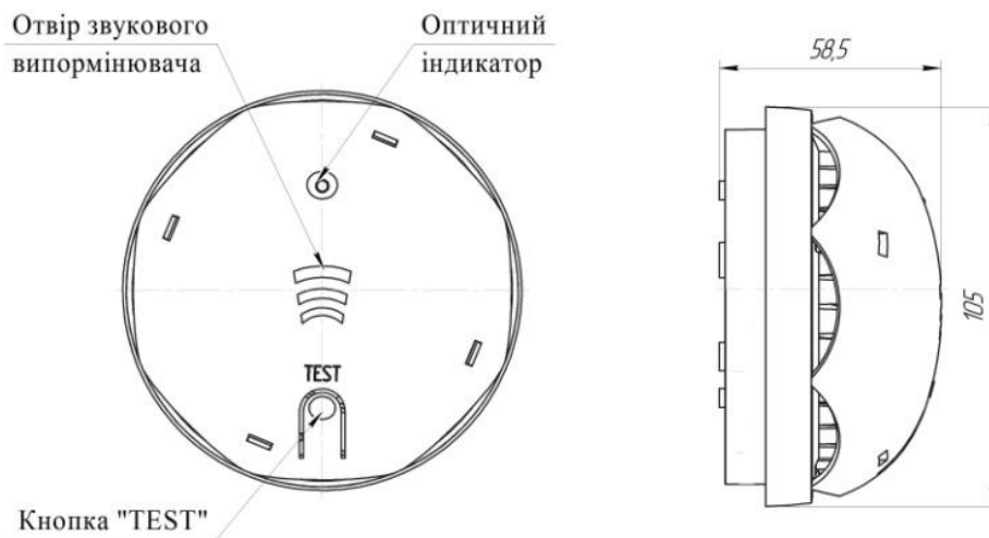
Малюнок 1- Загальний вигляд сигналізатора
