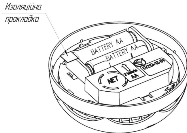
Малюнок 3 - Вилучення ізоляційної прокладки
