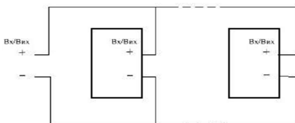
Малюнок 8 - Схема з'єднання сигналізаторів двопровідним шлейфом
